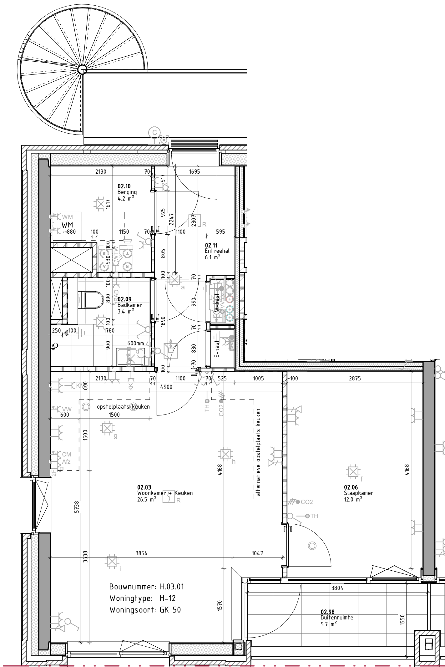
Bouwnummer H.03.01, H.05.01. Type H-12, 3e en 5e verdieping
