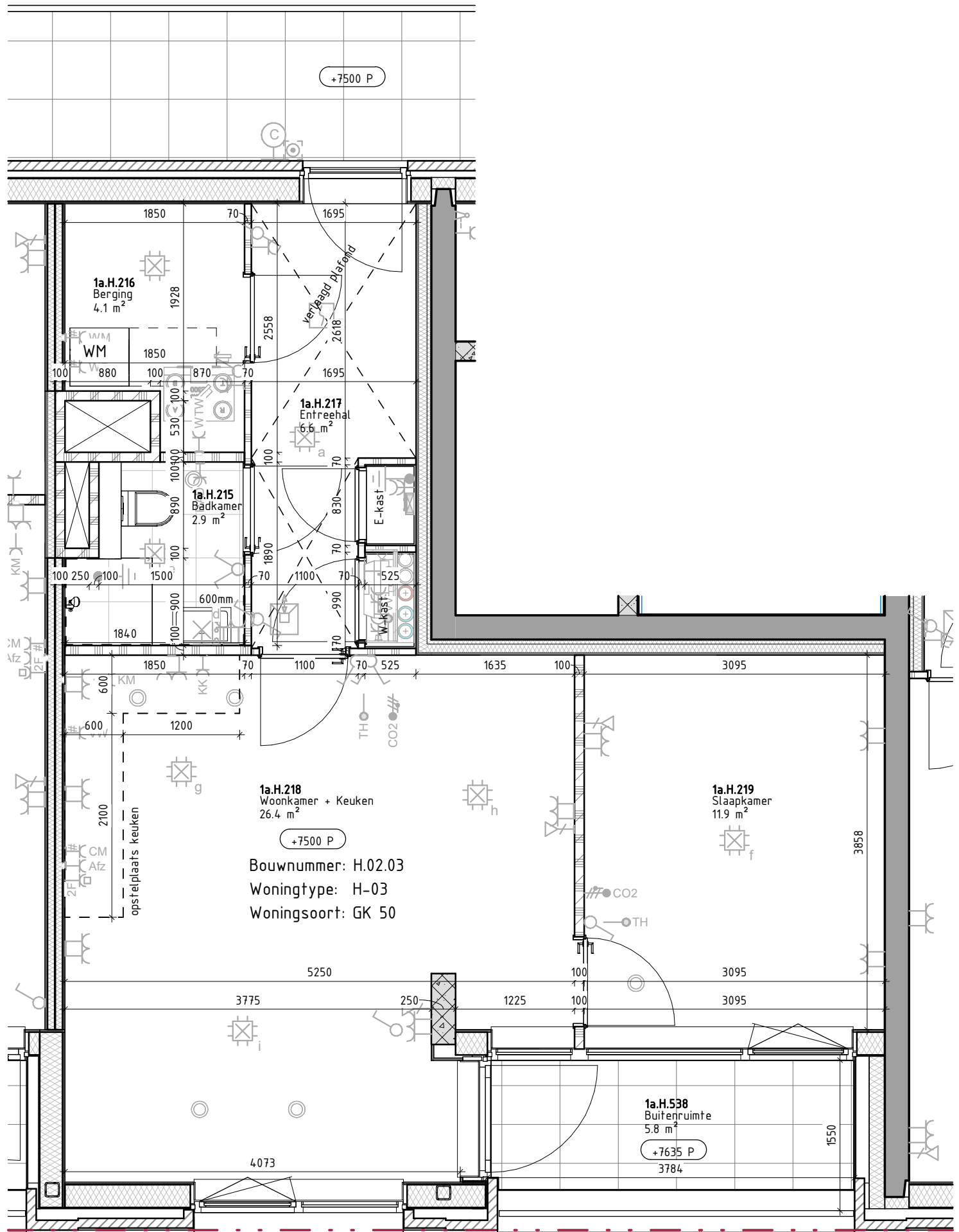
Bouwnummer H.02.03, Type H-03, 2e verdieping
