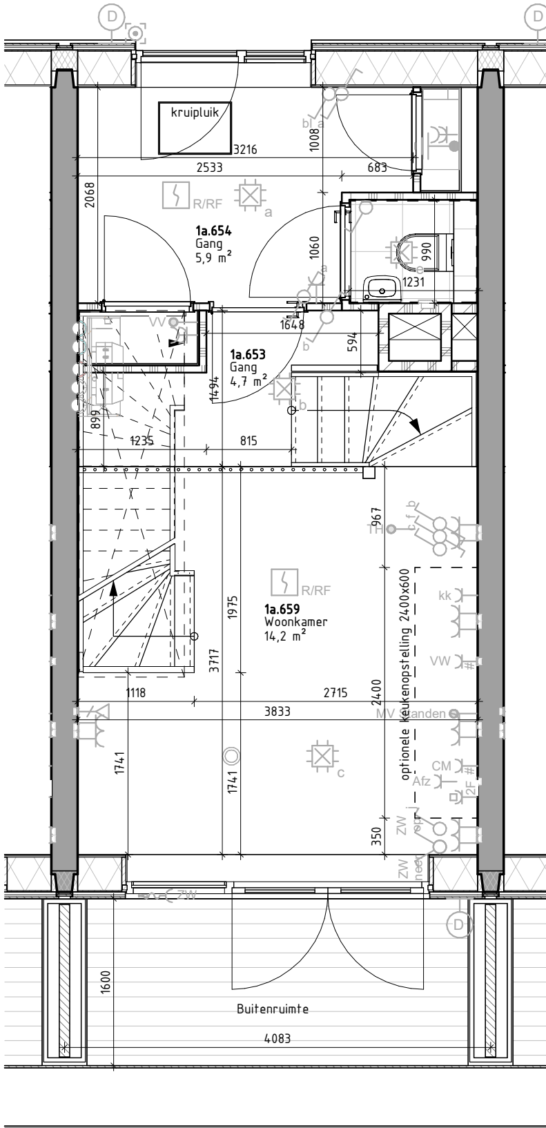
OPTIE Bouwnummer E.00.02 (Type E-01) Begane grond
